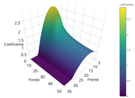
Fig. 13: Coeficientes de frente y fondo sin variables omitidas.
