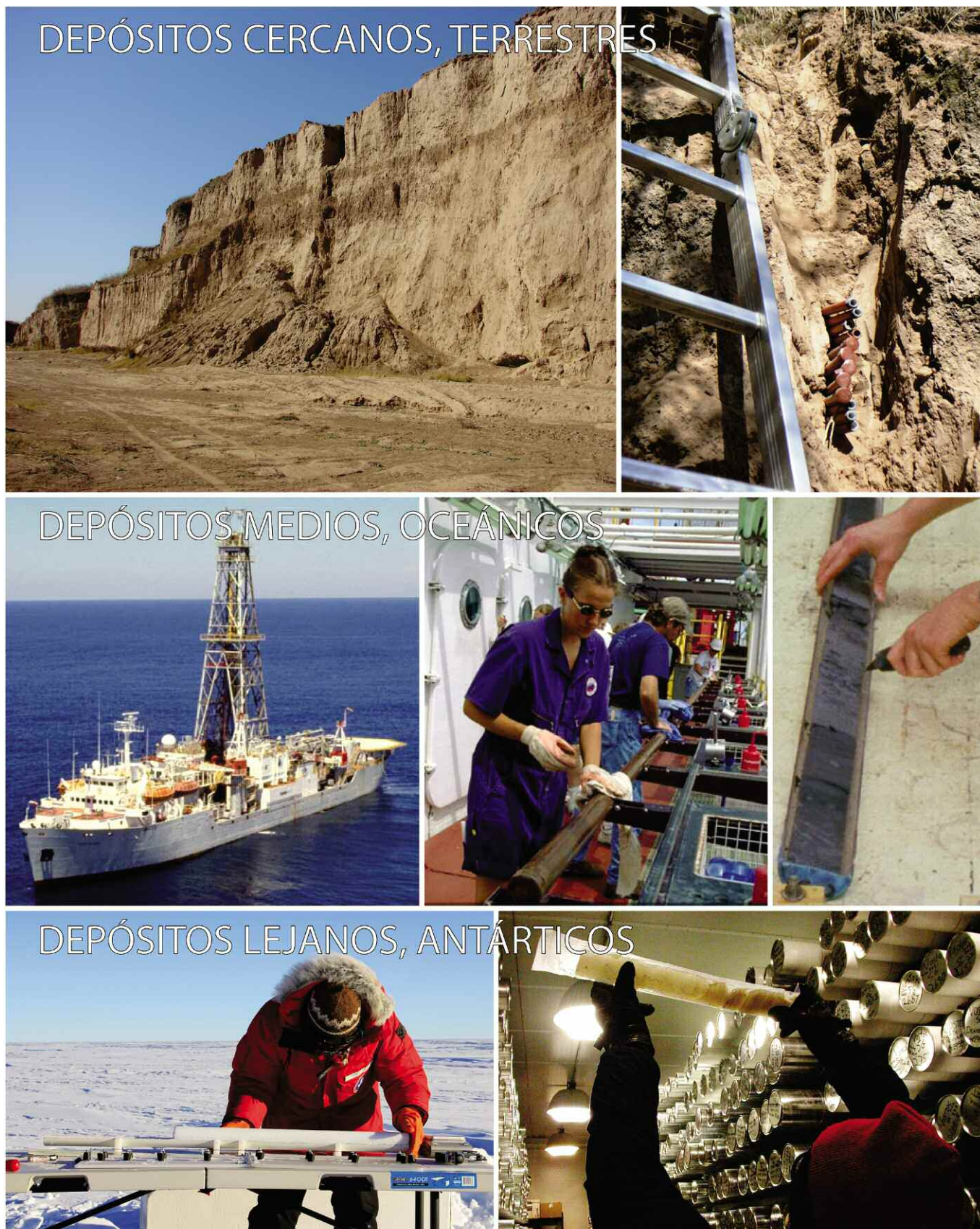
Figura 5. Ejemplos de distintos tipos de archivos climáticos. De arriba hacia abajo vemos: depósitos cercanos (loess), depósitos medios (océano) y depósitos lejanos (Antártida). A la derecha se ven los distintos tipos de muestras tomadas para cada tipo de archivo. Fuente de las fotos: IODP (Archivos oceánicos), British Antarctic Survey (Archivos antárticos).
